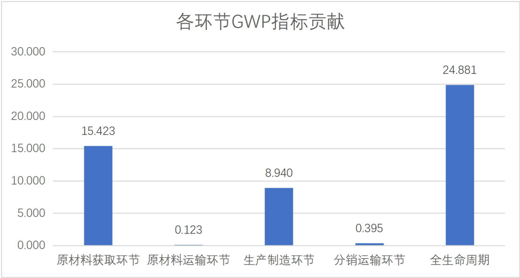
图 4.1 1 米冷热水聚丙烯管材（DN160）各环节的 GWP 指标贡献
