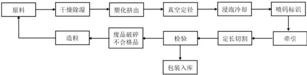
图 1.1 工艺流程图
